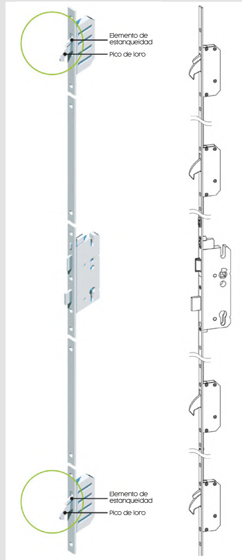
CERRADURA 3 PUNTOS
